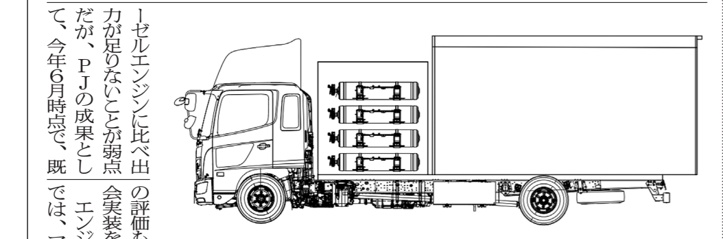
開発が進む水素エンジン搭載車のイメージ
